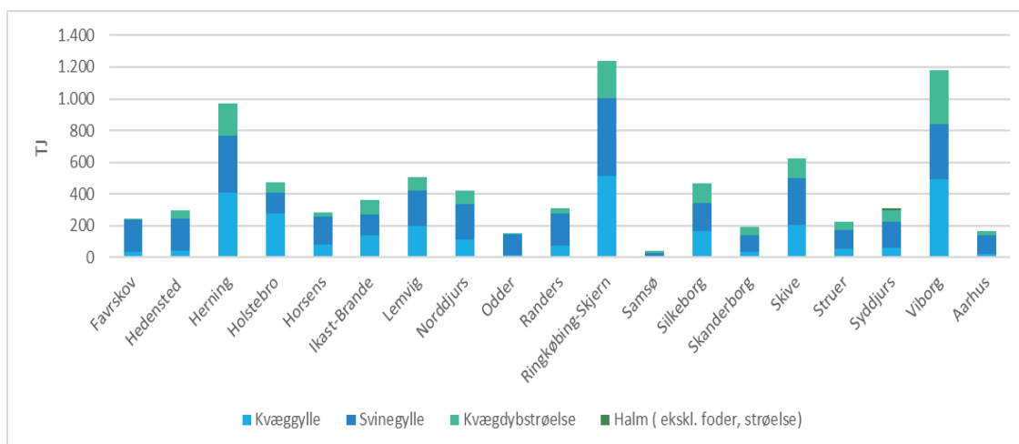
Figur 38 - Energipotentiale i biomasse til biogas ved 45 dages opholdstid, 100% udnyttelse af ressourcen
