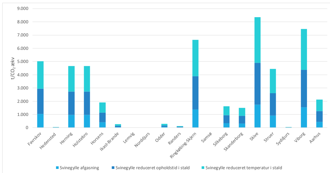
Figur 40 - Faktisk reduktion i CO 2 -ækv. ved leverance af svinegylle til biogas i 2018 og reduktionspotential ved gyllekøling og hurtig udsugning
