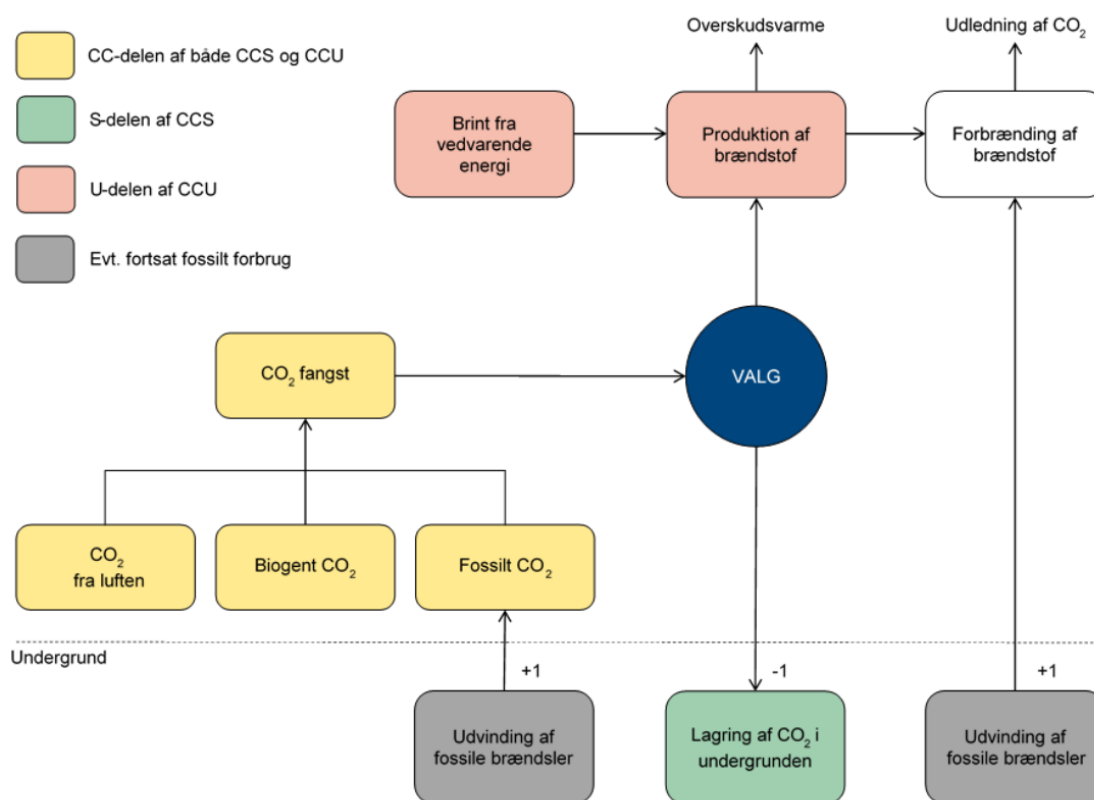
Figur 23 - Illustration af forskelle mellem CCS og CCU jf. Klimarådets rapport "Kendte veje og nye spor ti 170 pro-cents reduktion" Link
